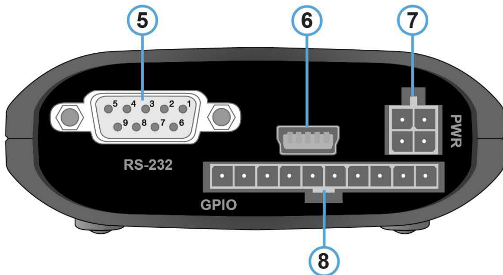
Рис. 2.2. Вид сзади
