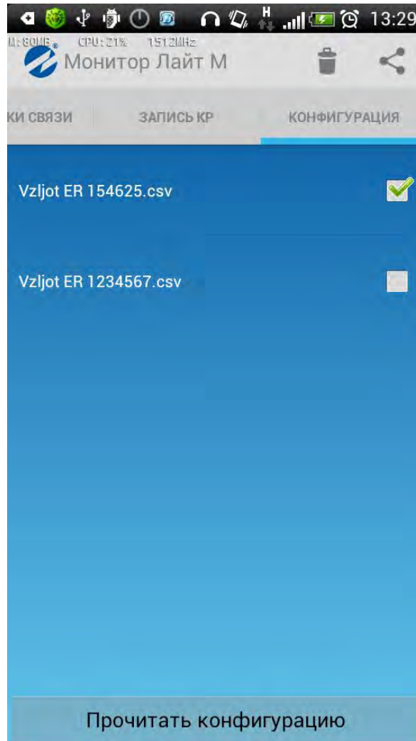
Рис.16. Вкладка «Конфигурация».
